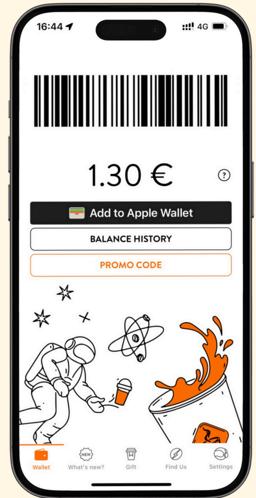
Caffeine
